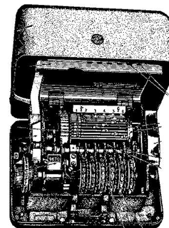
Figura 11. Mașina rotativă Enigma
